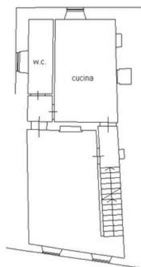
Piano Primo H. 3,04
