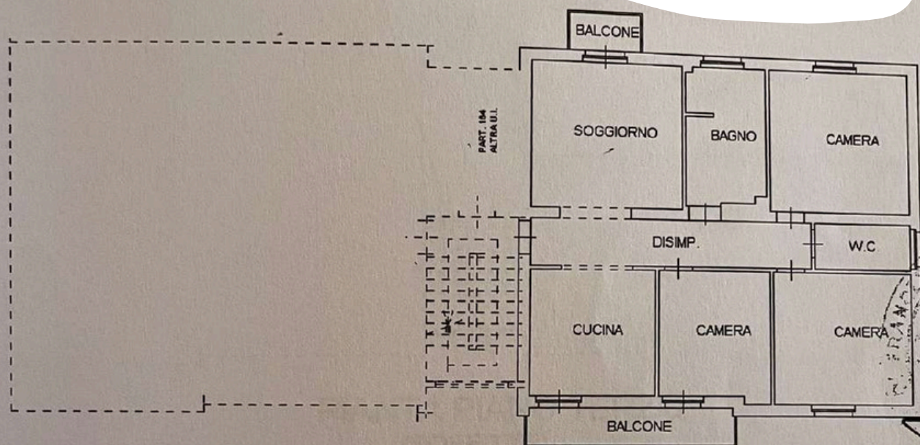
PIANTA PIANO PRIMO H=2,80 mt
