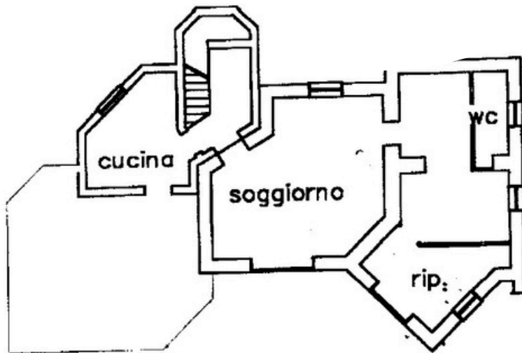
PIANO SOTTOSTRADA (SEMINTERRATO) H.MT.2.70
