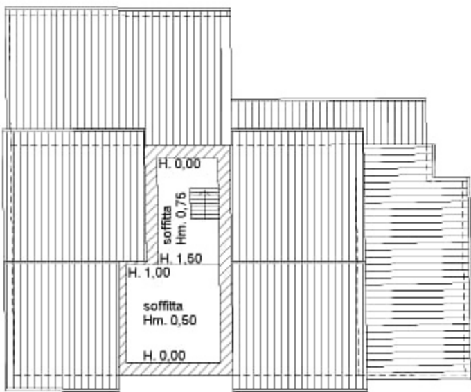
PIANTA SOTTOTETTO
